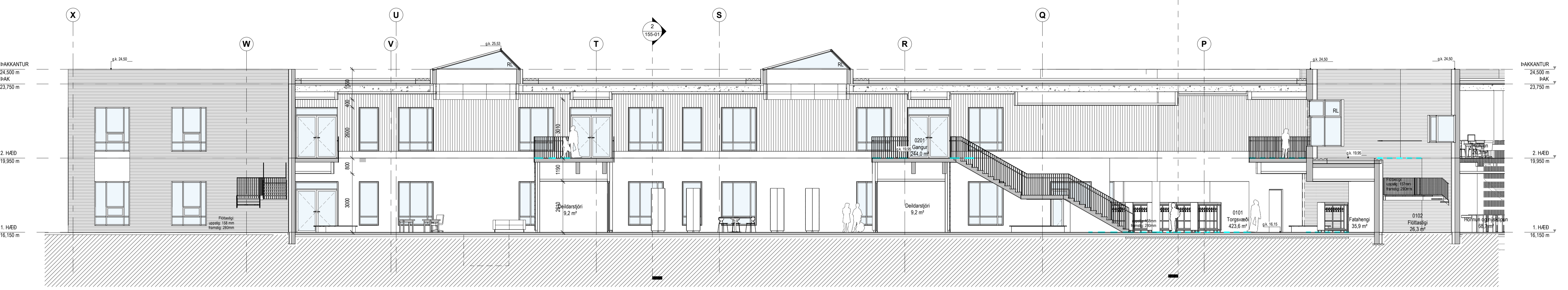
Á2 - Snið B 1 : 100
