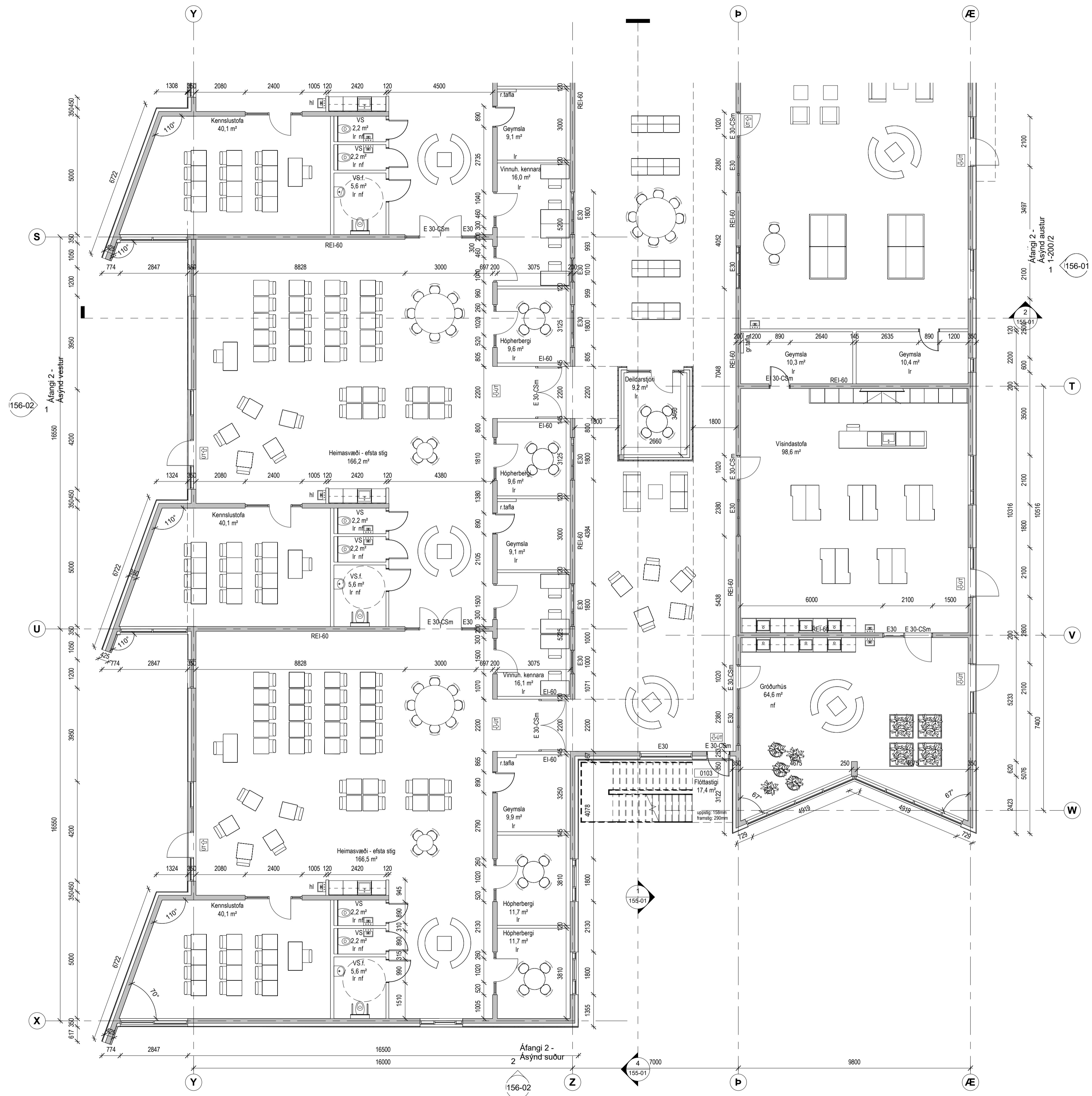
1. H/ÆD 1-100 Á2 - 2/2 1 : 100
