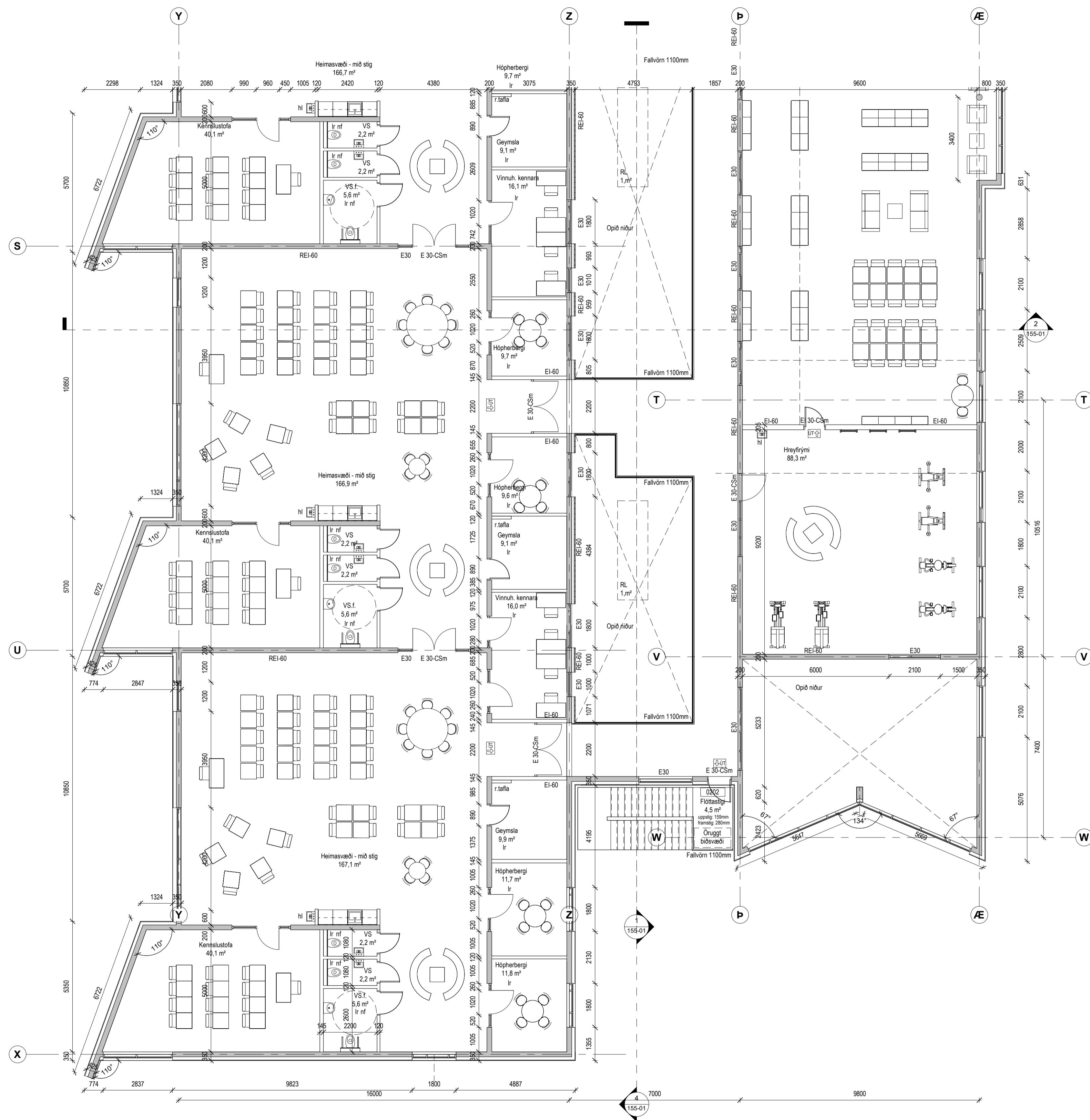
2. HÆÐ 1-100 Á2 - 2/2 1: 100
