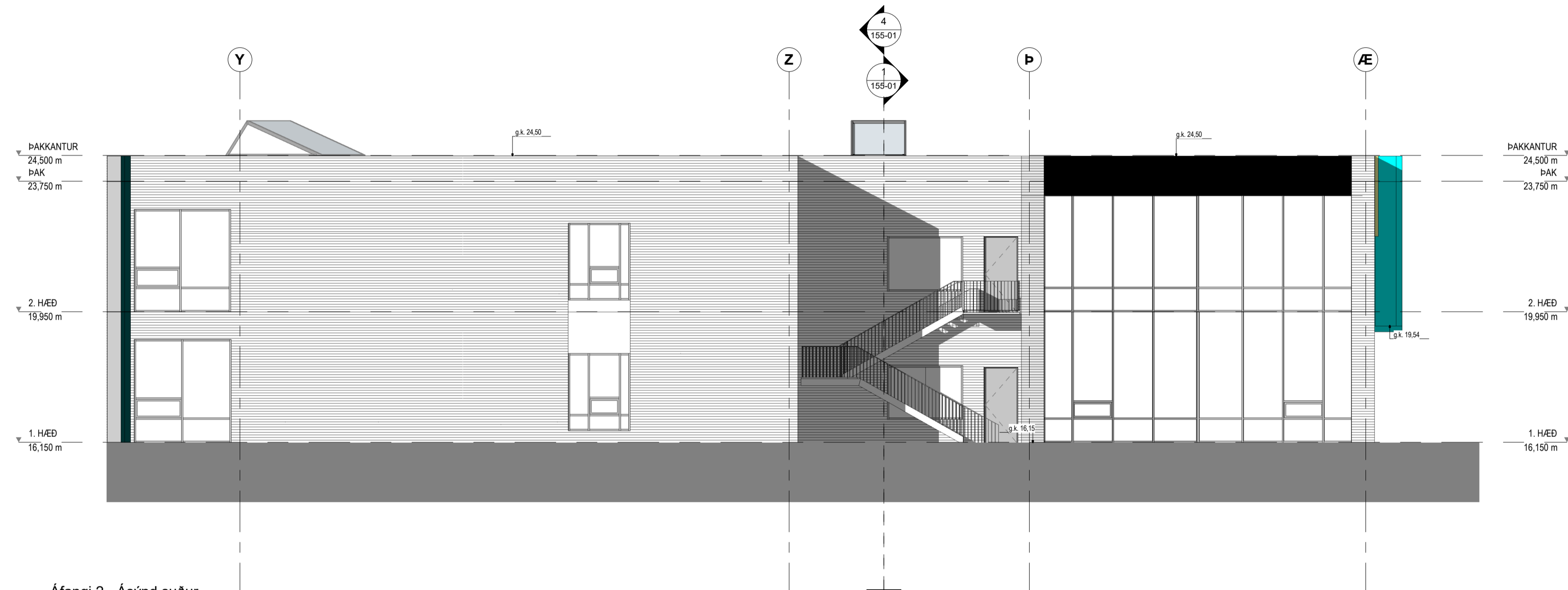
Áfangi 2 - Ásýnd suður 1 : 100
