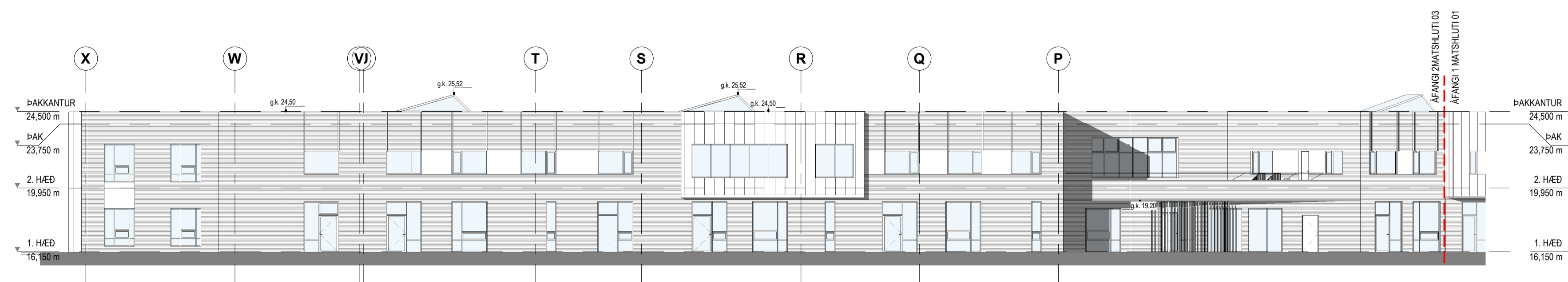
Áfangi 2 - Ásýnd austur 1-200 1 : 200
