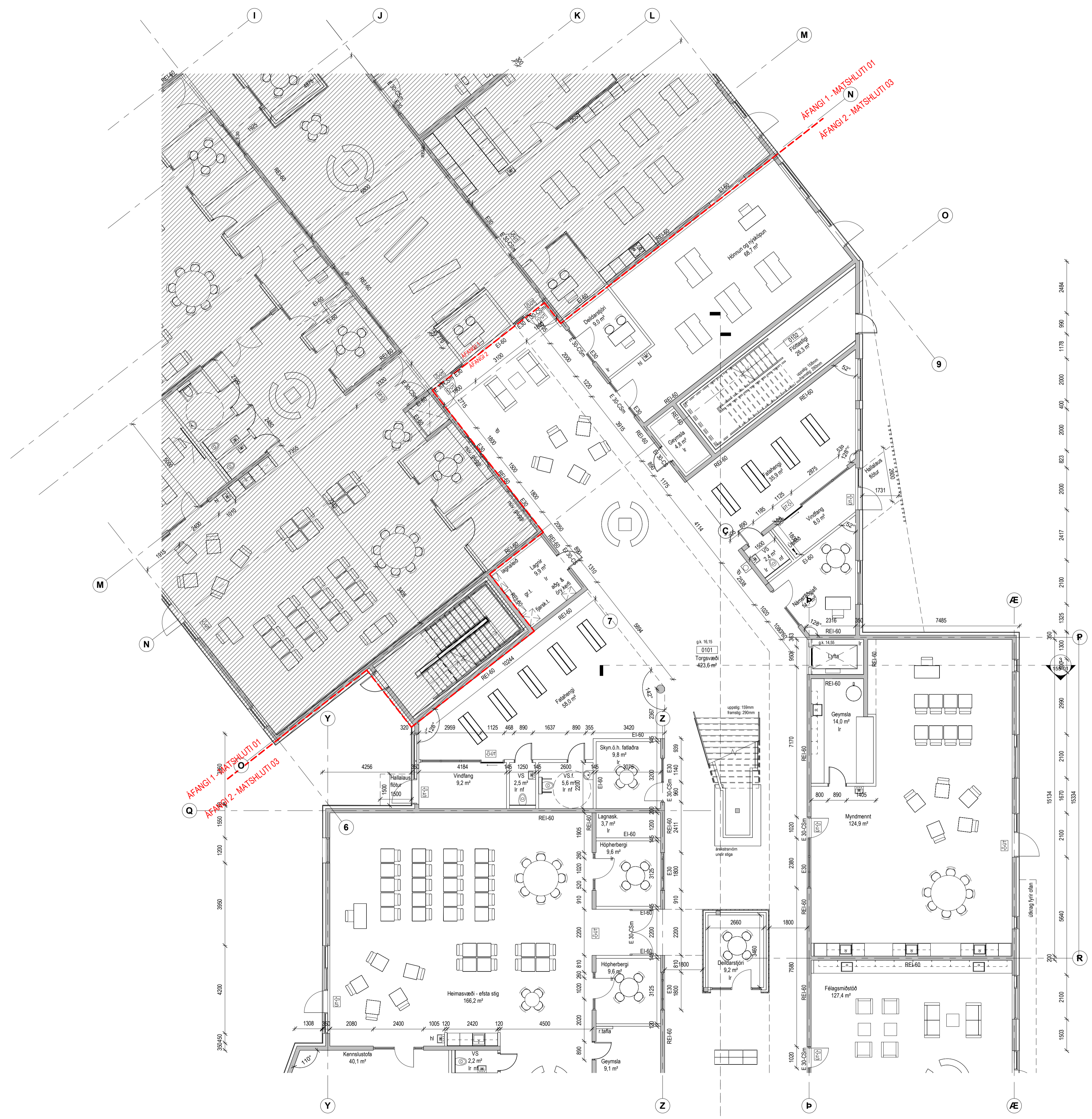
1. HÆÐ 1-100 Á2 - 1/2 1: 100
